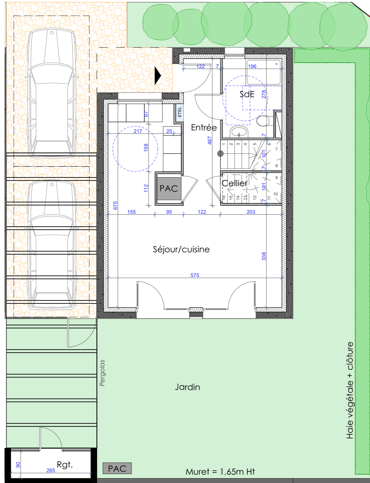
NIVEAU REZ DE CHAUSSEE
